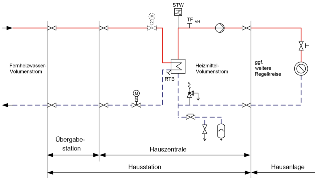
Abbildung 12: Hauszentrale-Raumheizung Prinzipschaltbild für den indirekten Anschluss
