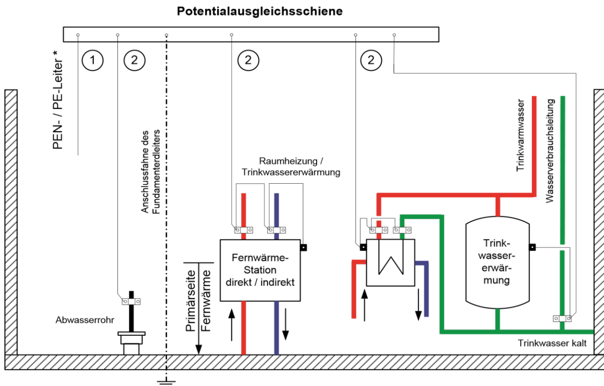
Stromversorgers Abbildung 4: Beispiel eines Potentialausgleichs
